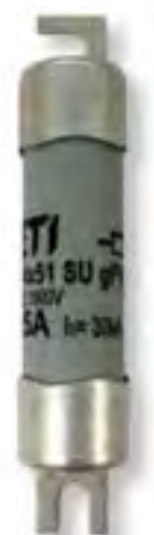
Type SU Contacts
