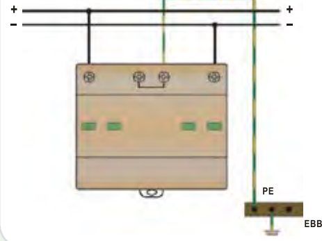
Y configuration ETITEC S B-PV U/I_{imp} Y
