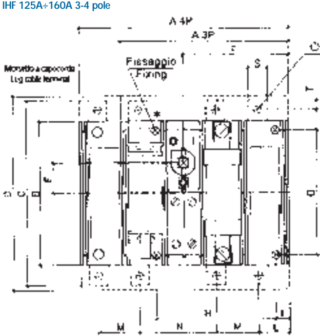
IHF 125A÷160A 3-4 poli IHF 125A÷160A 3-4 pole
