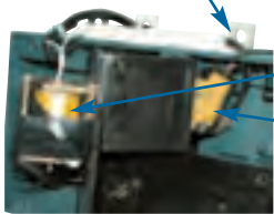
connessioni a capocorda lug cable terminals
