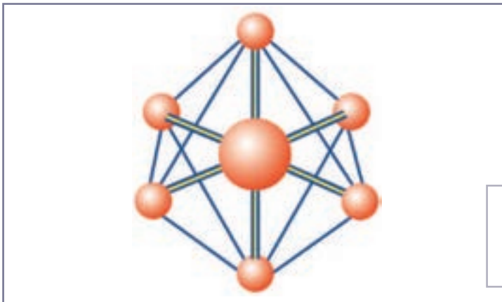
FIG. 2 STRUTTURA MOLECOLARE DEL SF 6 SF 6 MOLECULAR STRUCTURE
