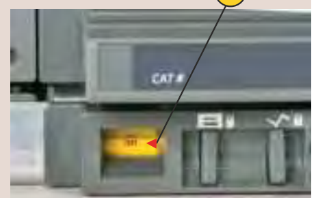
Fig. 1.12: Circuit Breaker in Maintenance Position Abb. 1.12: Leistungsschalter in Wartungsstellung Fig. 1.12: Interruttore in posizione di Manutenzione
