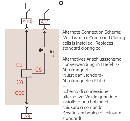
Connection scheme Command Closing Coil BLOCK A Anschlussschema Befehls-Abbrufmagnet BLOCK A Schema di connessione della bobina di chiusura a comando Morsettiere A
